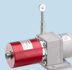
Capteur à câble (0 à 1250 mm)
